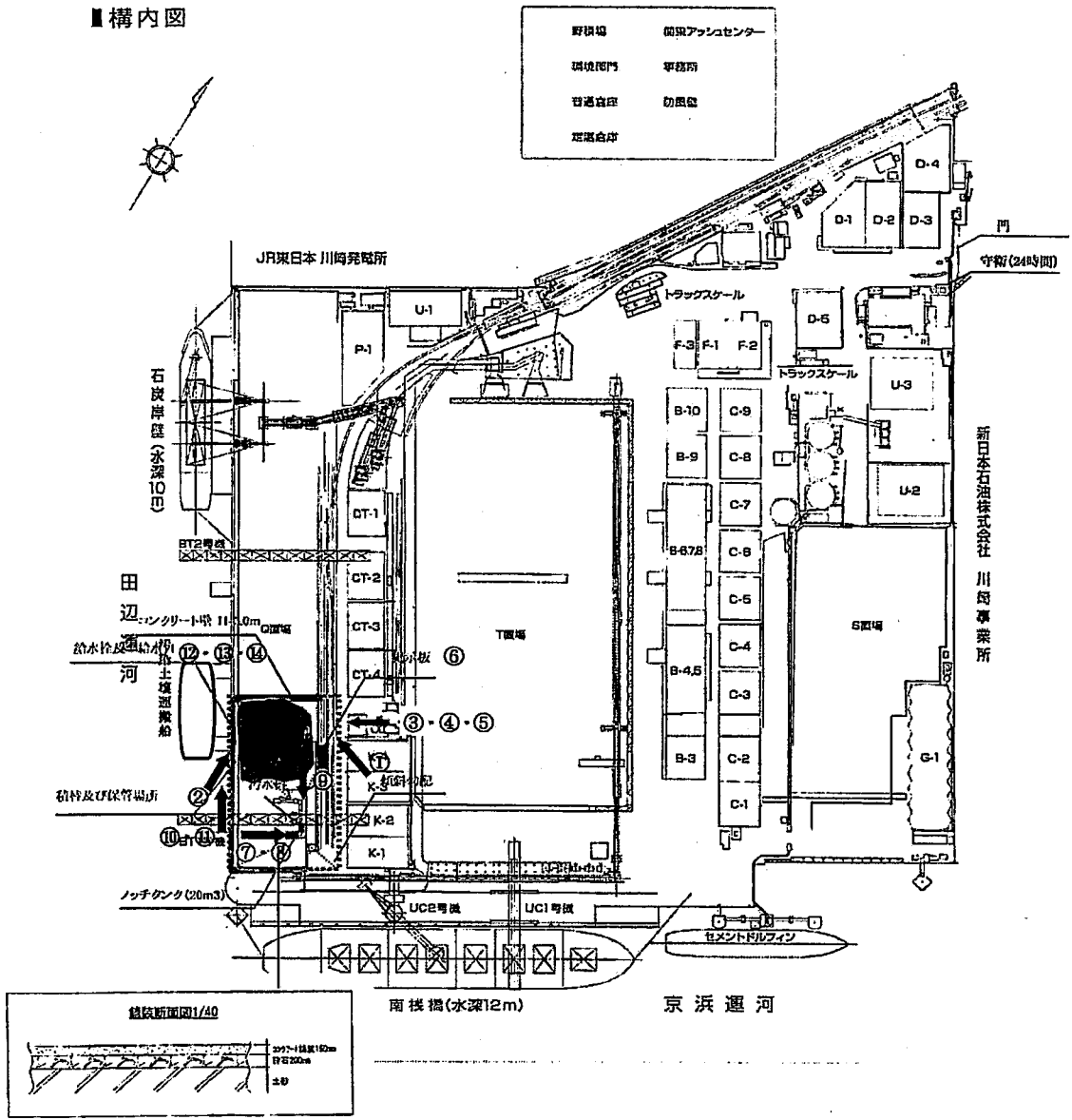
■ 構内図
