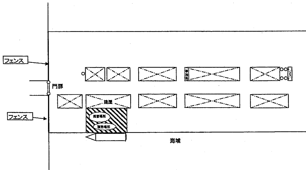
積替・保管場所拡大図
