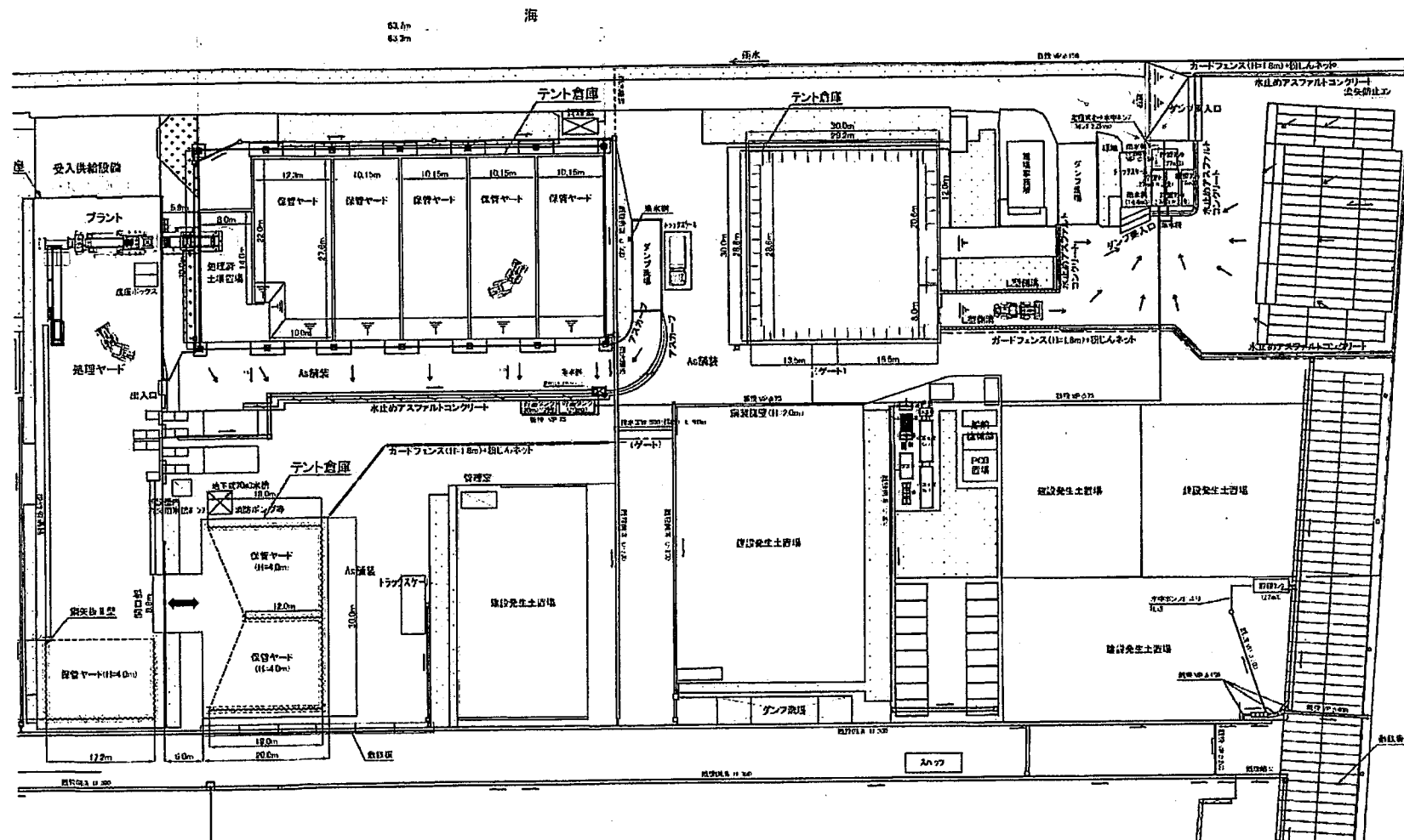
③排水経路図
