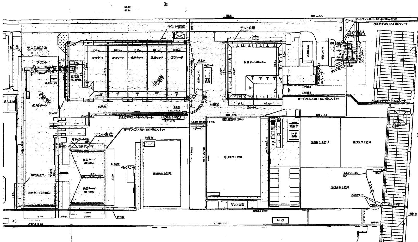
②床面舗装位置図
