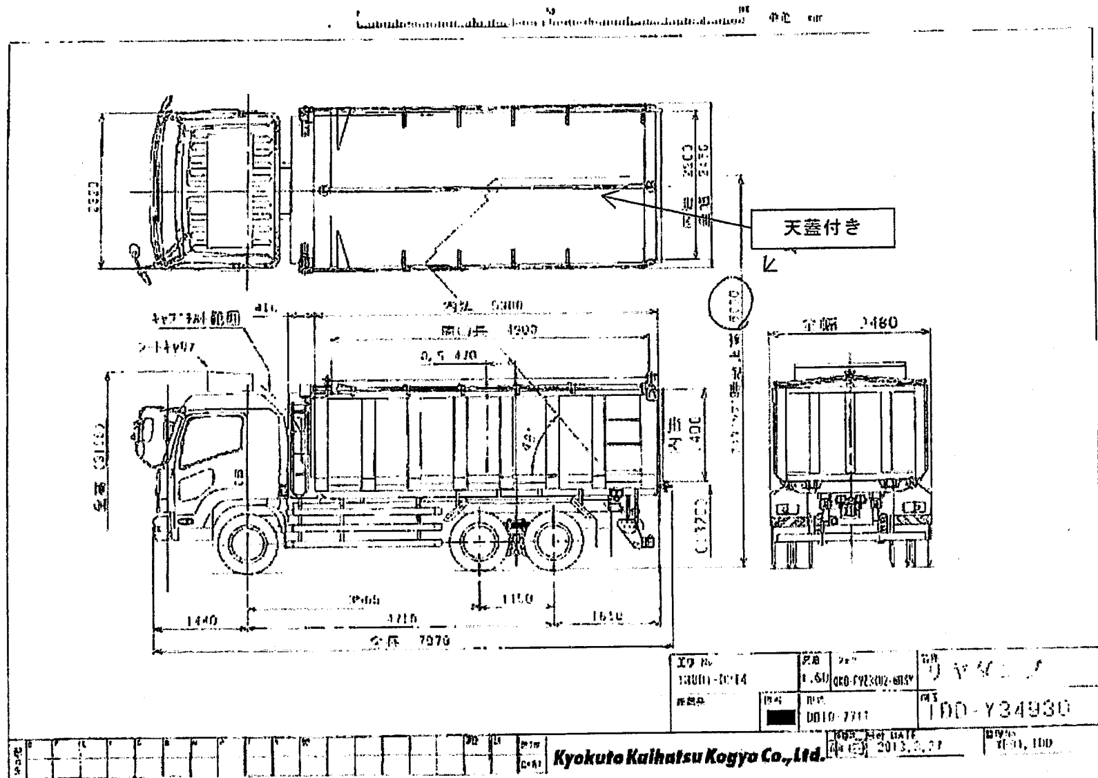
図 3-3 天蓋付きダンプトラック（運搬車両）の構造図
