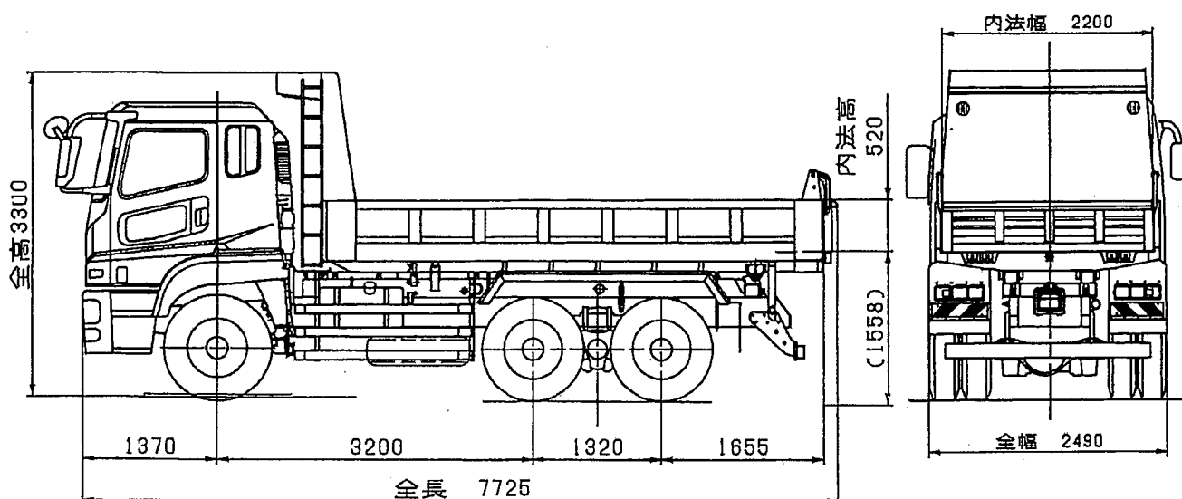
運搬車両構造図（ダンプトラック）
