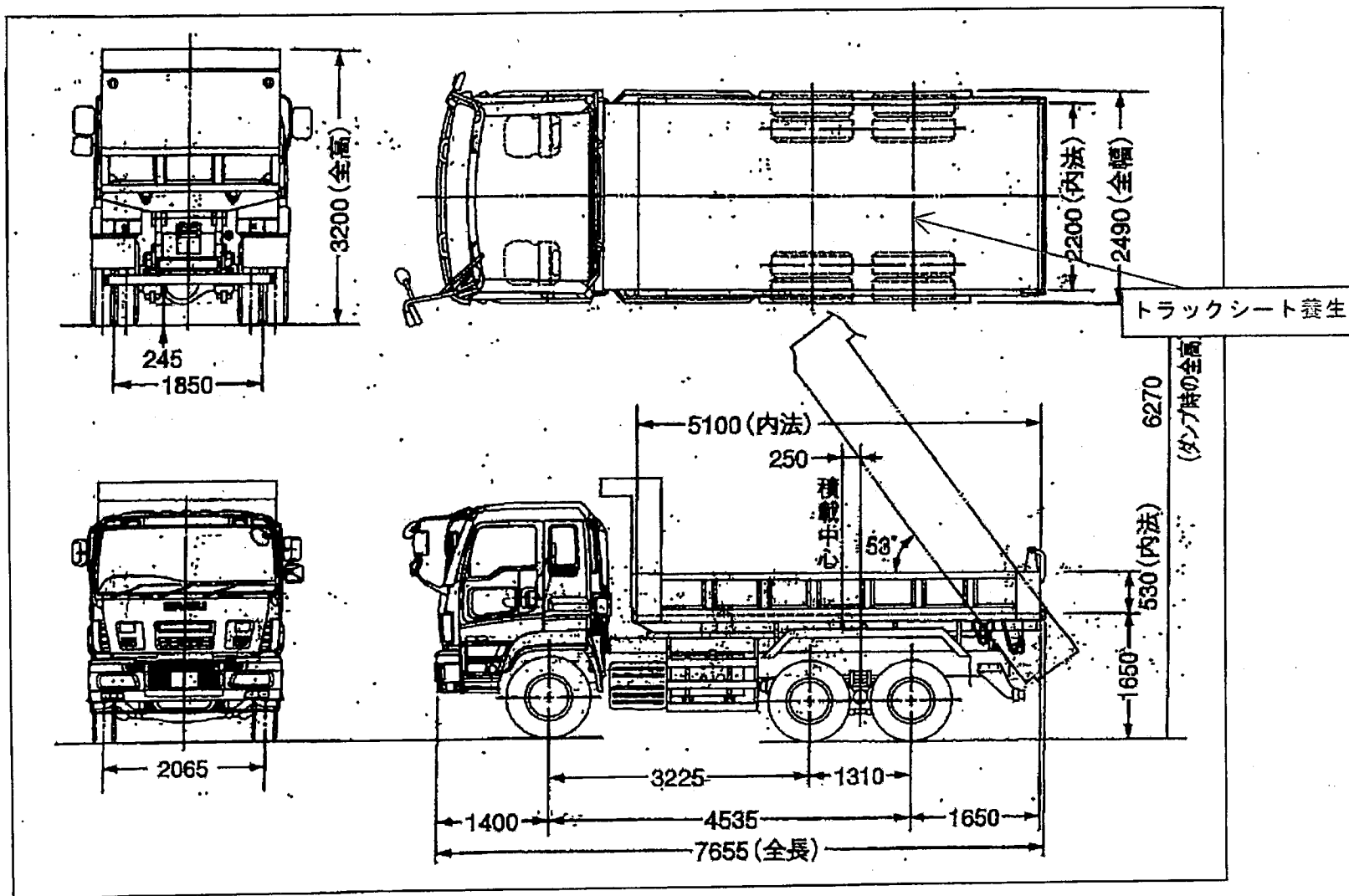
図 3-2 ダンプトラック (運搬車両) の構造図
