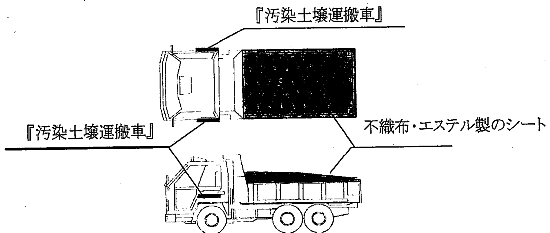
図 3-1 運搬車両の養生 (ダンプ車による運搬の場合)
