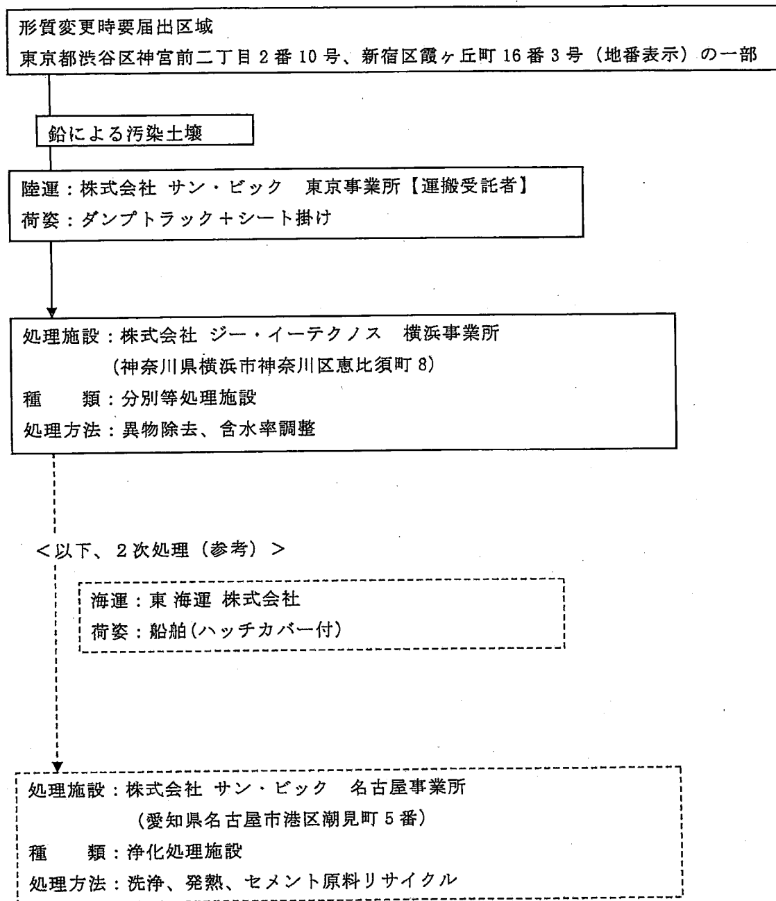
図 2-1 汚染土壌の運搬フロー図
