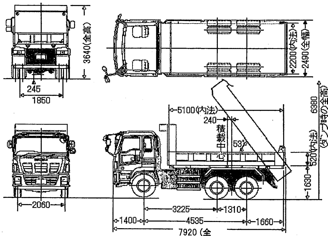
運搬車輛 構造図
