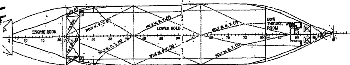
船舶構造図
