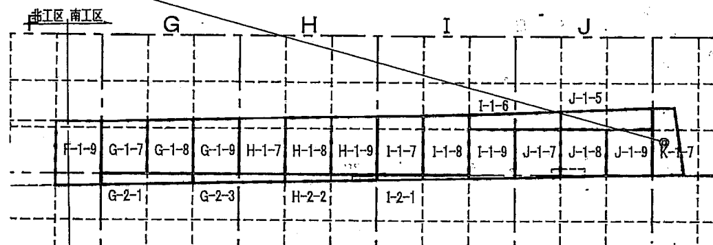
平面図 (B部)
