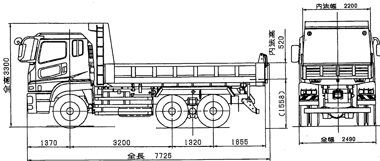
運搬車両構造図 (ダンプトラック)
