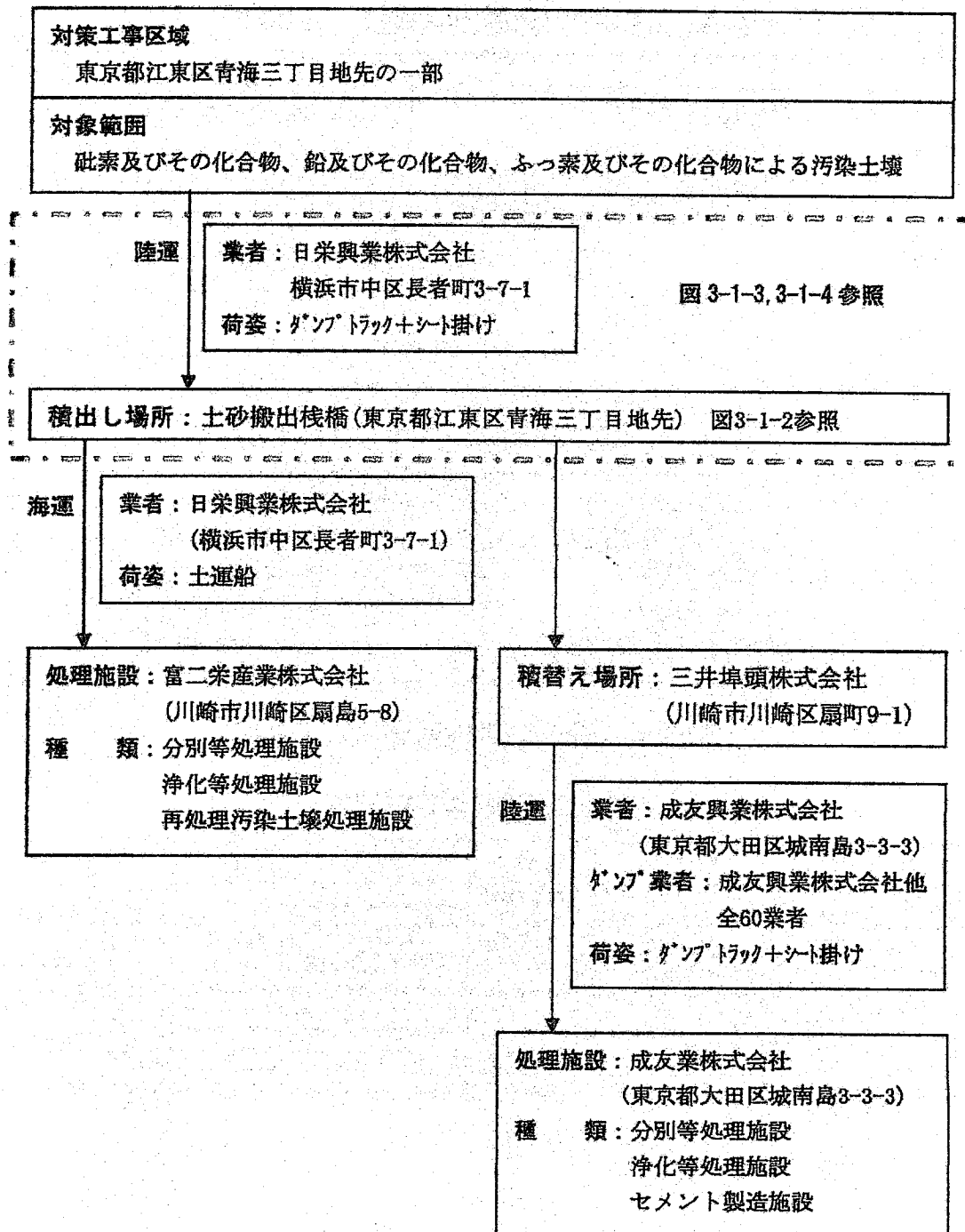
図 3-1-1 汚染土壌海上運搬を含むフロー図
