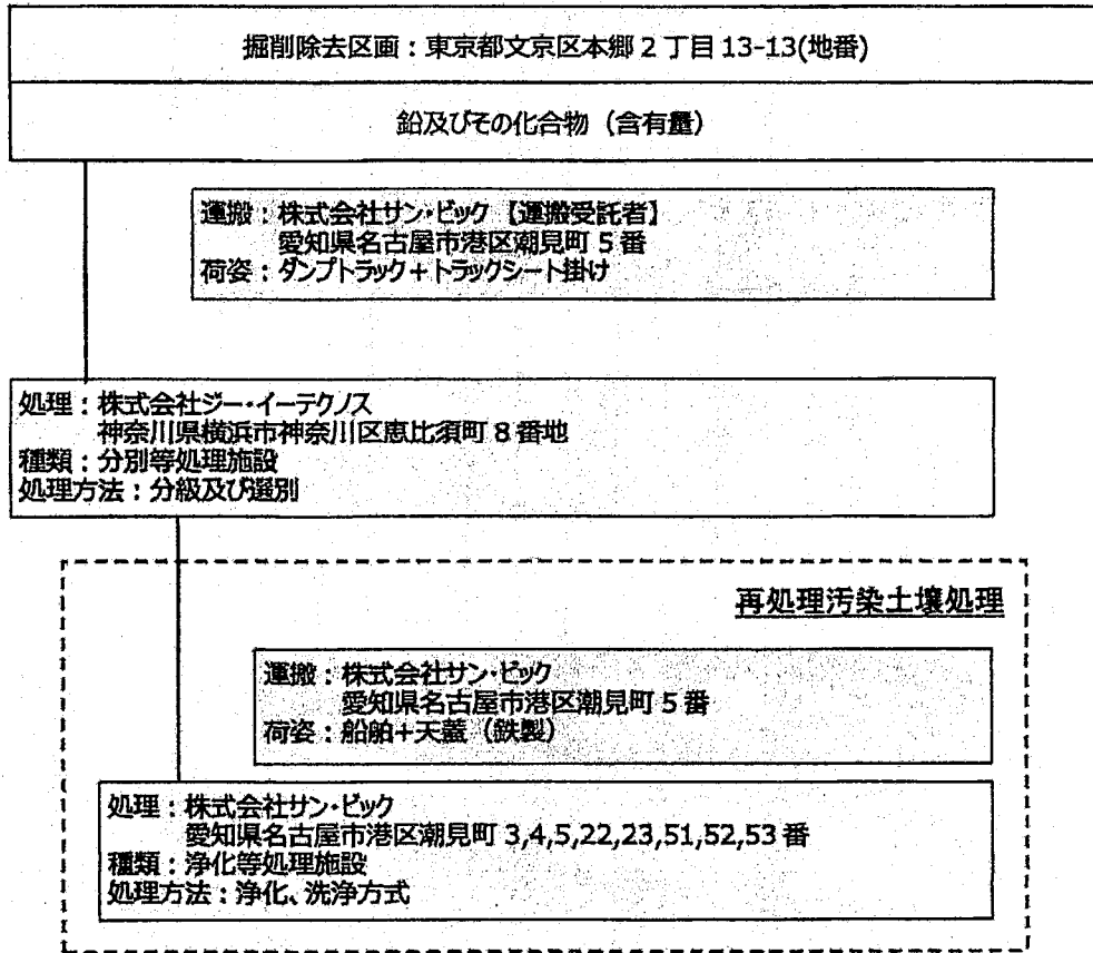
図 1-1 汚染土壌運搬処理フロー図
