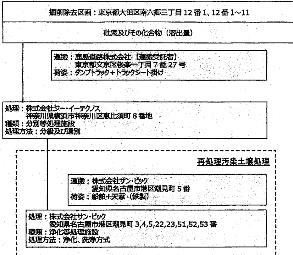
図 3-1 汚染土壌運搬処理フロー図
